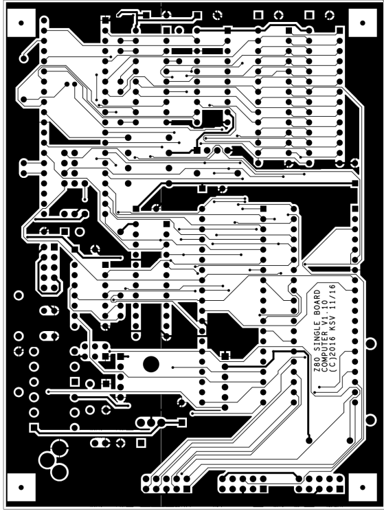
BOTTOM Clad
